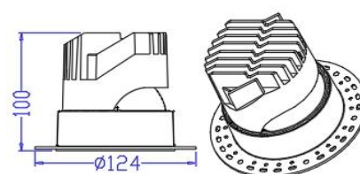
Trimless
